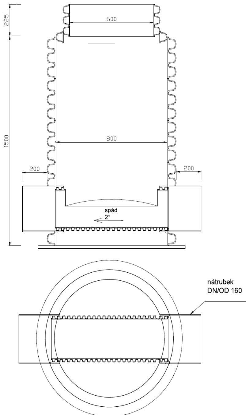
základní provedení šachty, celková výška 1,7m
